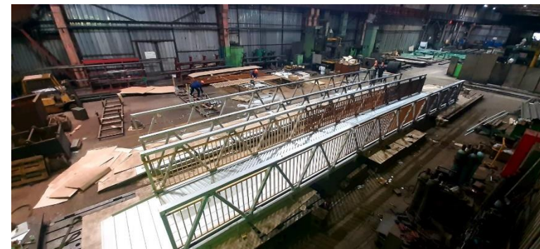
Стапель для контрольной и окончательной сборки
