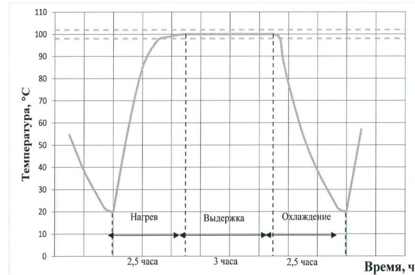
Рис. 2. Диаграмма полного цикла "нагрев-выдержка-охлаждение" образца кабеля при температуре (100\pm 2)\text{ }^{\circ}\text{C} .
