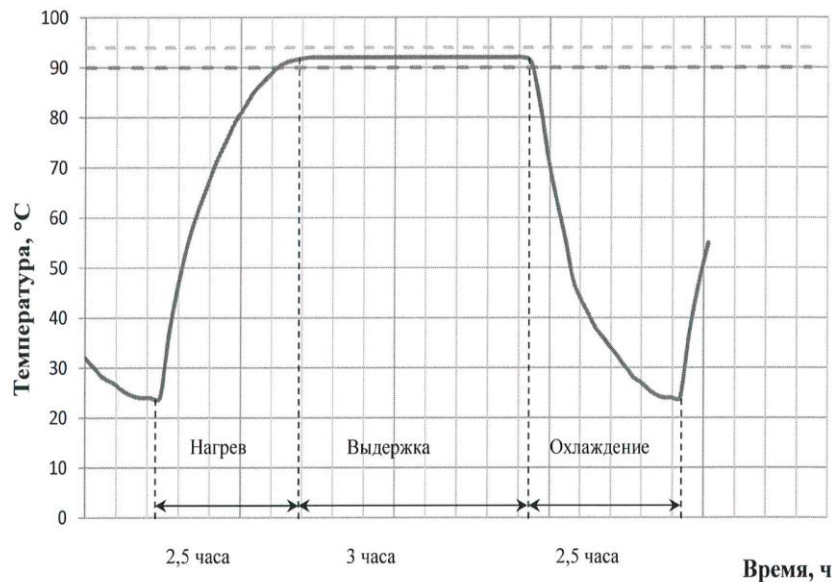
Рис. 1. Диаграмма полного цикла "нагрев-выдержка-охлаждение" образца кабеля при температуре (92\pm 2)\text{ }^{\circ}\text{C} .
